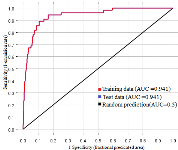
图 1 模型适用性检验的 AUC 值 Fig. 1 AUC value of model suitability test
