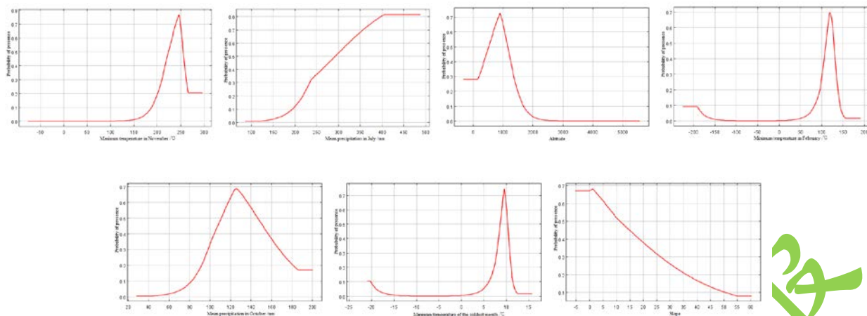
图 6 云南省小粒咖啡的主导环境因子与地理分布概率的关系
