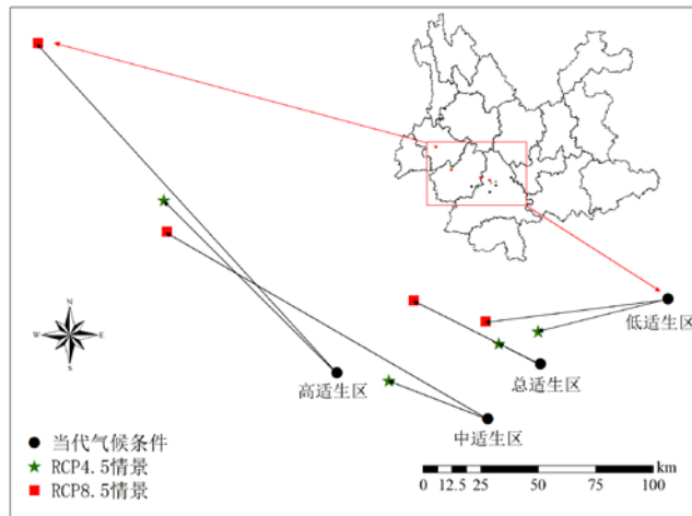
图5 云南省小粒咖啡适生区在不同气候情景下的质心变化
