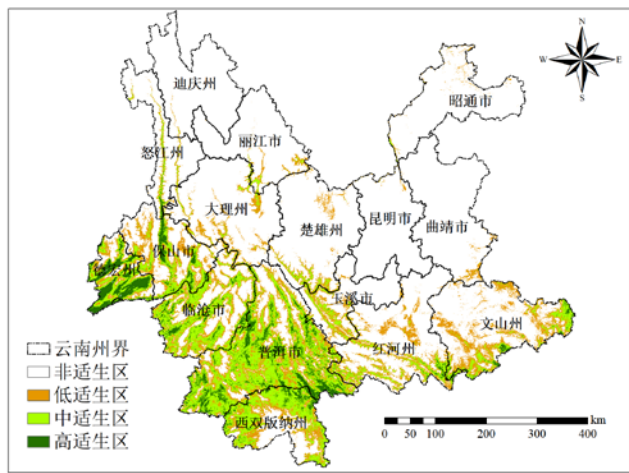
图 2 当前气候条件下云南省小粒咖啡适生区分布
