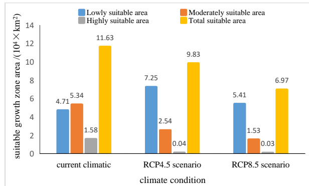
图 4 不同气候情景下小粒咖啡在云南的适生区分布变化
