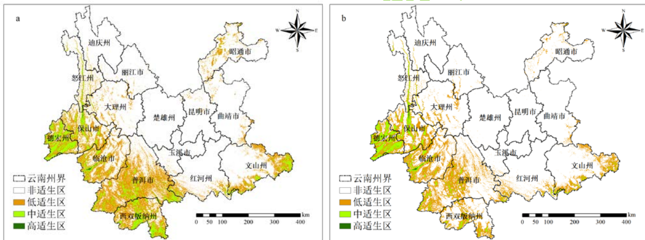
图 3 RCP4.5 (图 a)、RCP8.5 (图 b) 气候情景下小粒咖啡在云南的适生区分布图
