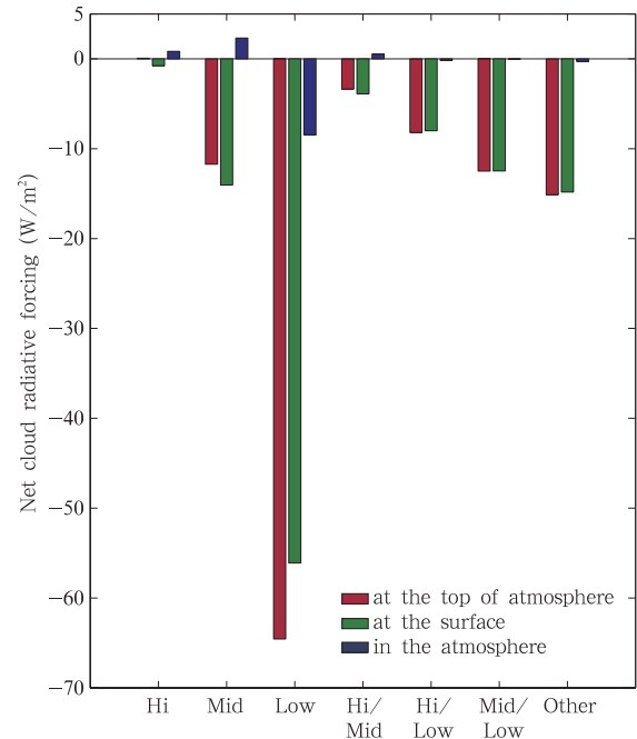
图2 大气层顶、地表以及大气中不同类型云的区域年均净云辐射强迫
