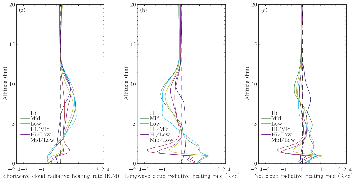
图4 不同类型云区域年平均云辐射加热率廓线
