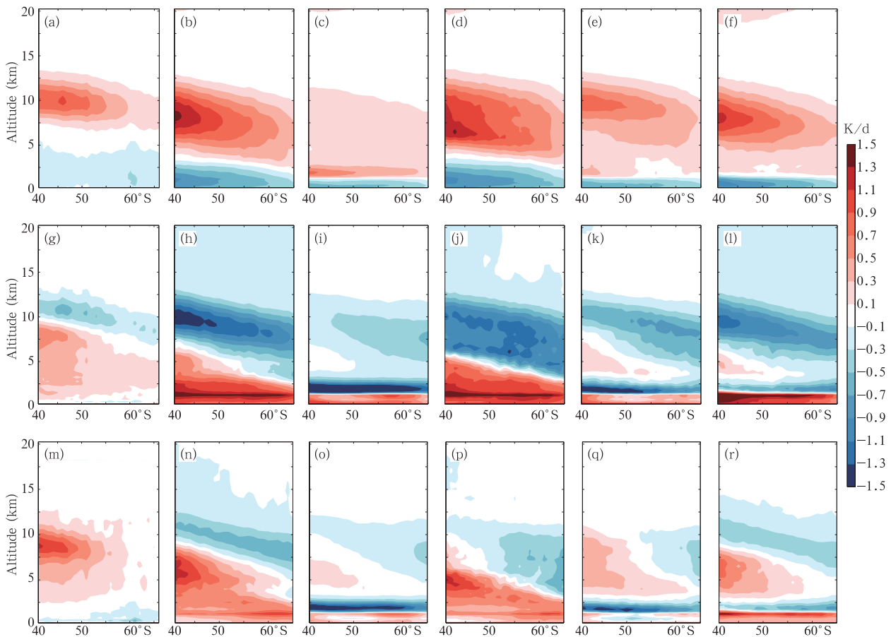
图 3 不同类型云的辐射加热率廓线的纬向分布
