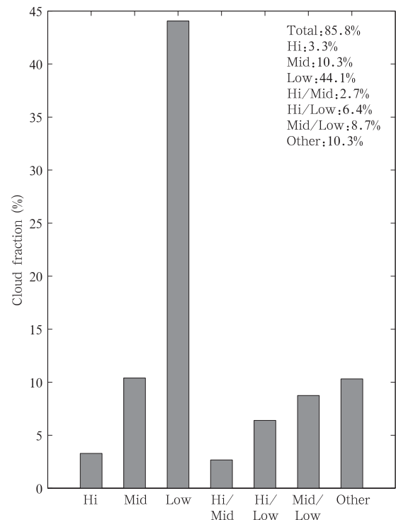
图 1 研究区域高云(Hi)、中云(Mid)、低云(Low)、高云/中云(Hi/Mid)、高云/低云(Hi/Low)和中云/低云(Mid/Low)的区域年均云量
