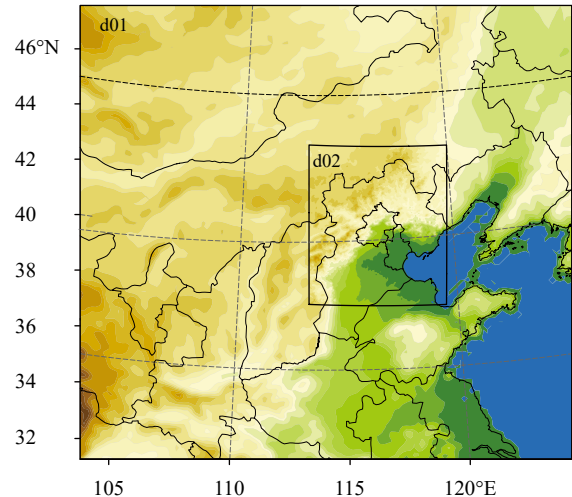
图 1 模式区域设置
