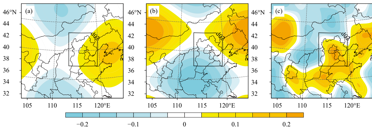
图 2 不同 SPPM 试验对 MYNN 边界层参数化方案参数随机扰动的水平形态 (a. SPPM_Meso, b. SPPM_025, c. SPPM_L150)
