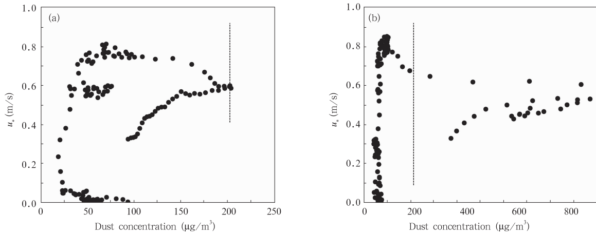
图 3 2004年3月16日(a),27日(b)浑善达克沙地两次沙尘天气过程中沙尘浓度与摩擦速度的关系
