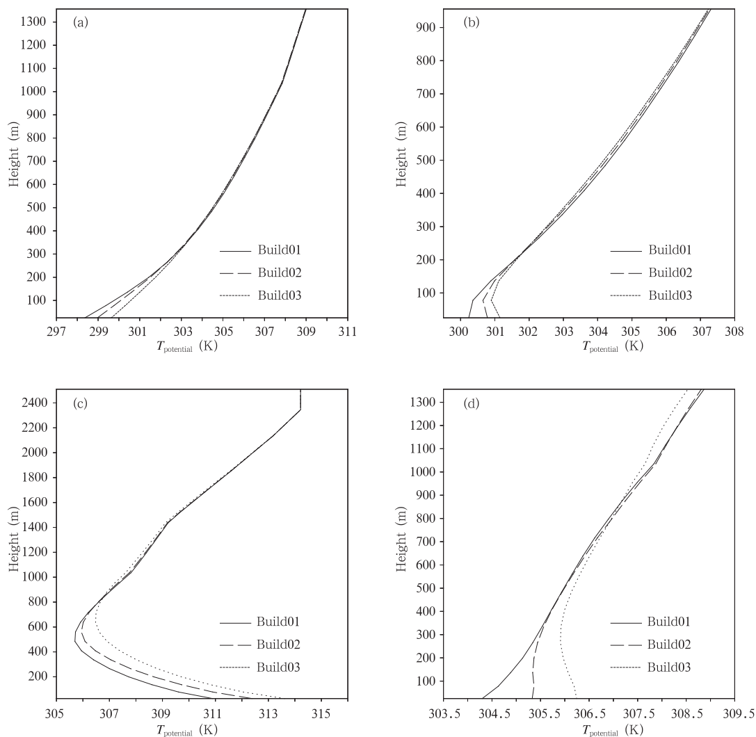
图 6 城市面积扩张对不同时刻位温廓线的影响(a. 02 时, b. 07 时, c. 14 时, d. 20 时)
