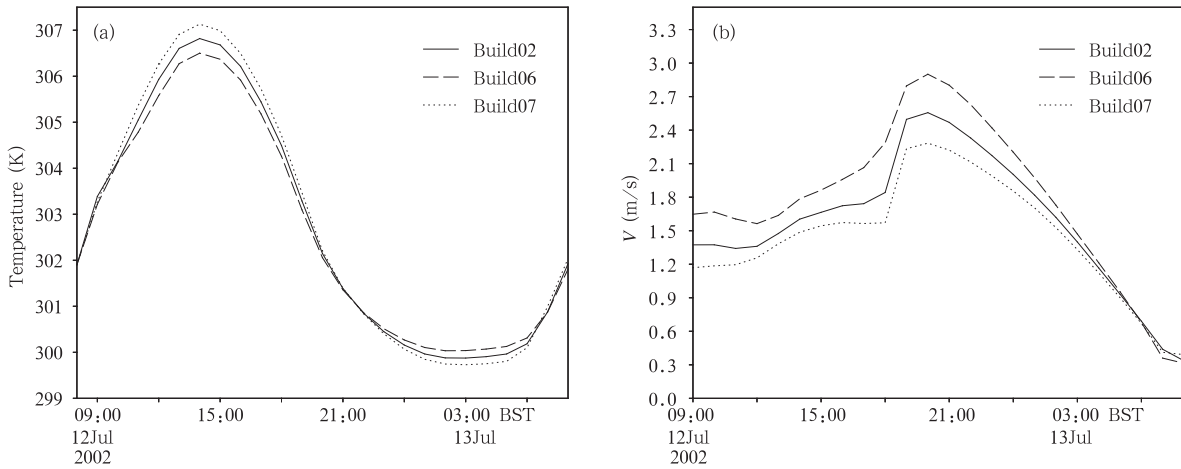
图 10 建筑物分布密度变化对城市地面气温和风速的影响 (a. 气温, b. 风速)
