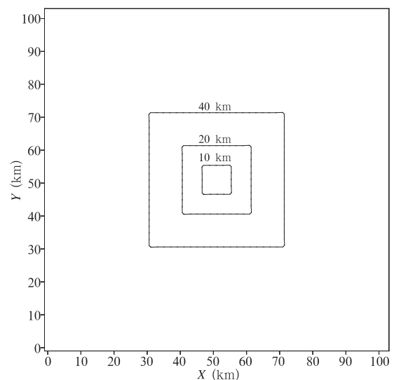
图3 敏感性试验模拟域示意图分别代表不同面积的城市范围
