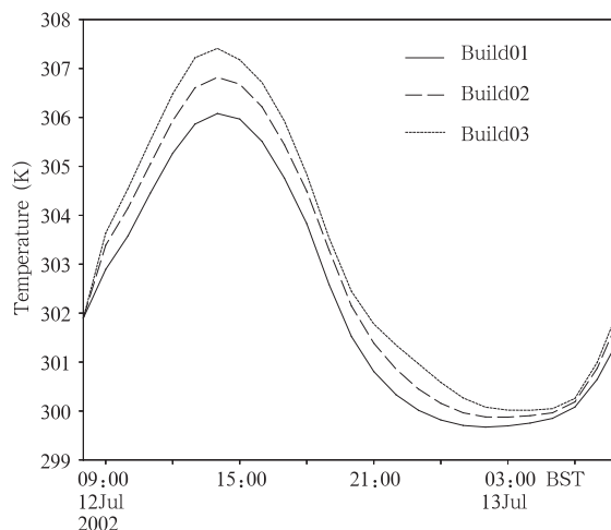
图 4 城市面积扩张对城市气温的影响(单位:K)
