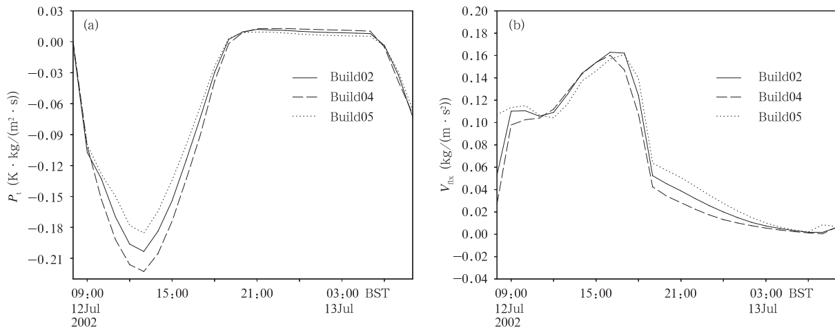
图 9 城市建筑物高度变化对城市平均热量通量、动量通量的影响 (a. 热量通量, b. 动量通量)
