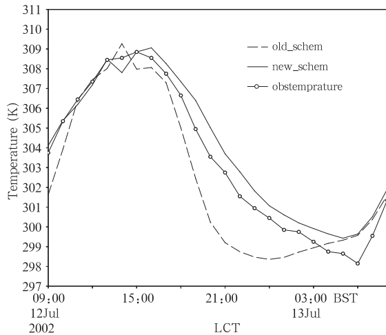
图2 地面气温模拟结果与观测资料对比(单位:K)
