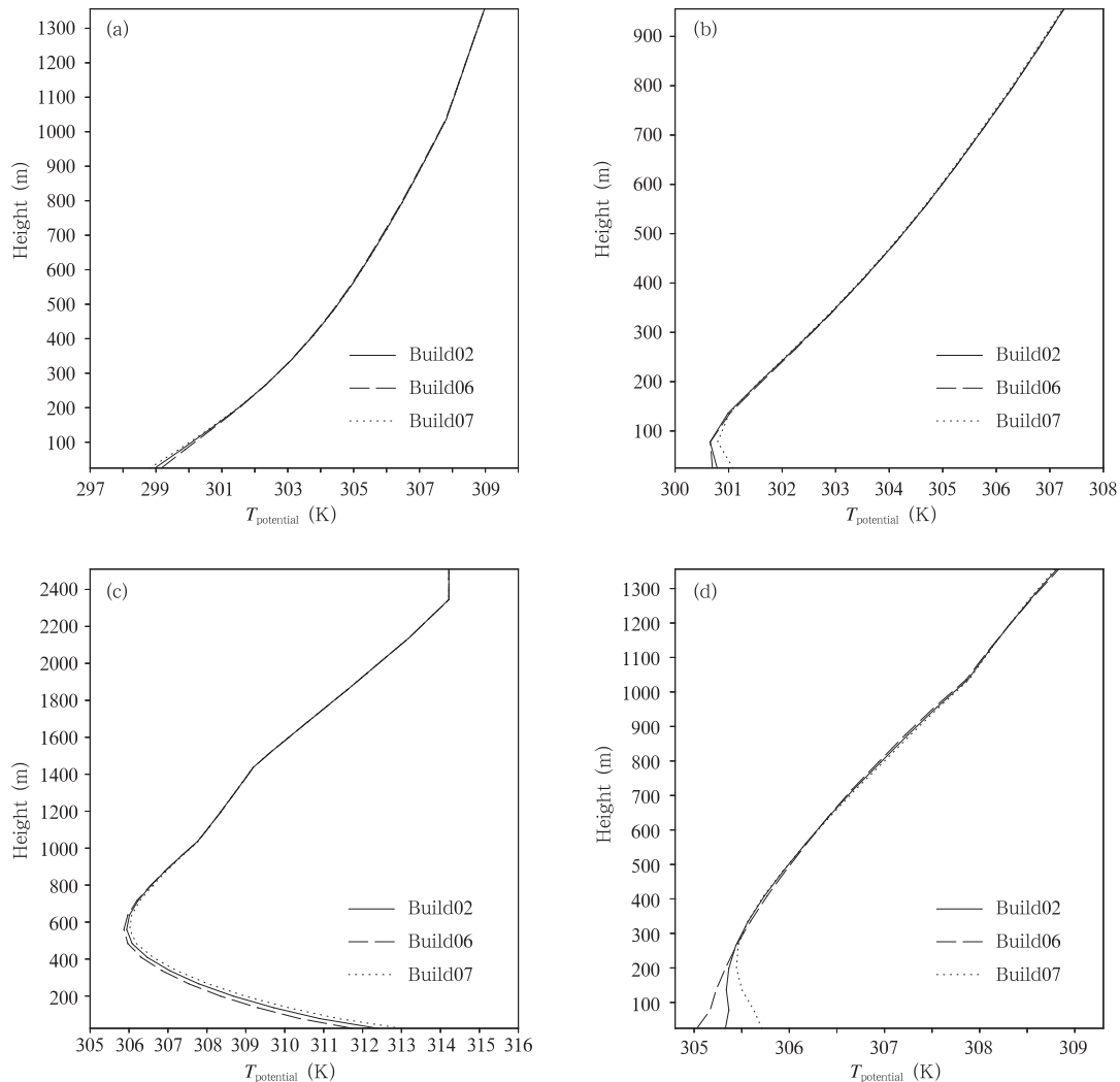
图 12 建筑物分布密度变化对不同时刻城市位温廓线的影响 (a. 02 时, b. 07 时, c. 14 时, d. 20 时)
