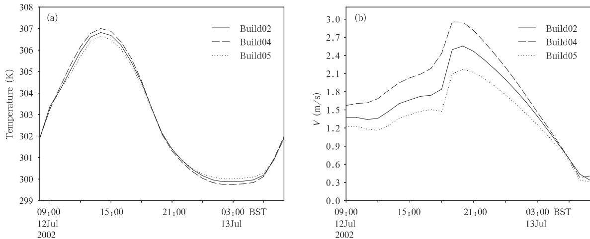
图 8 城市建筑物高度变化对城市地区地面气温和风速的影响 (a. 气温, b. 风速)
