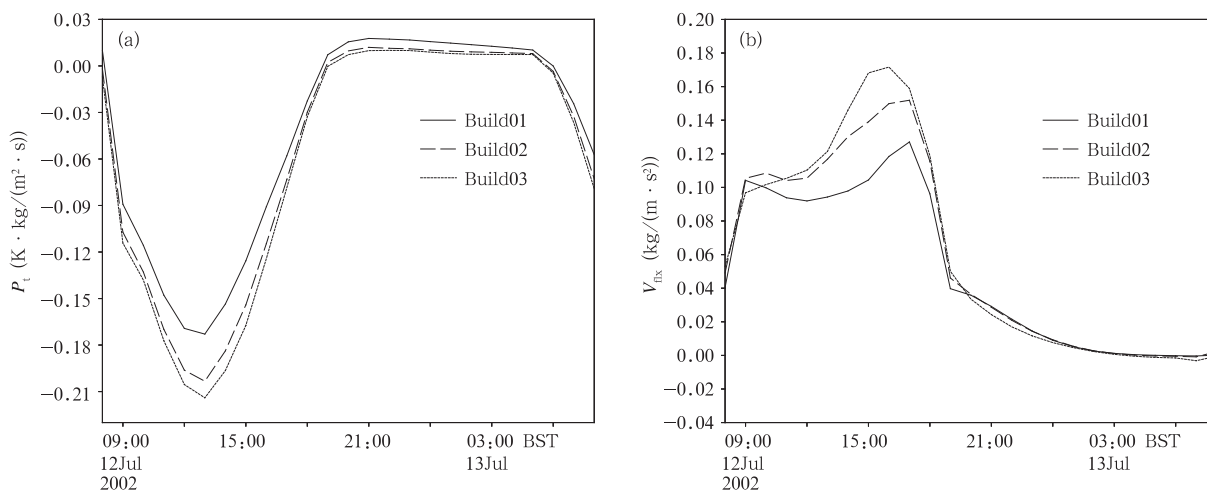
图 5 城市面积扩张对城市热量通量和动量通量的影响 (a. 热量通量, b. 动量通量)
